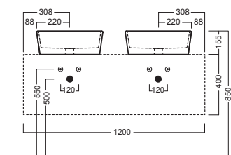
SLIDING wood system_taglio 4 doppio - cut 4 double
